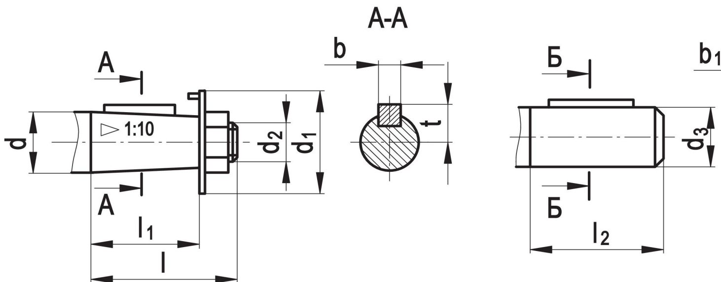
Варианты сборки редуктора ВК-475
