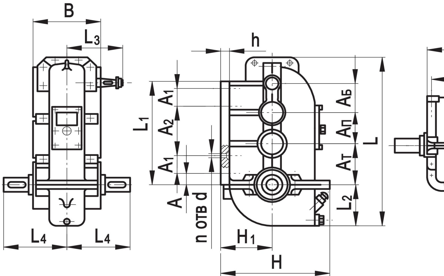
Редуктор ВК-475 Размеры и диаметр входного и выходного вала ВК-475 А 65 А 60 А 210 ВХОДНОЙ Выходной
