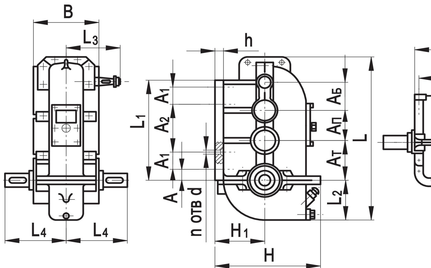
Редуктор ВК-550 Размеры и диаметр входного и выходного вала ВК-550
