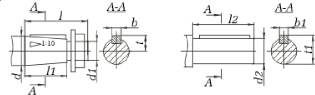
Редуктор ВК-550 Размеры и диаметр входного и выходного вала ВК-550
